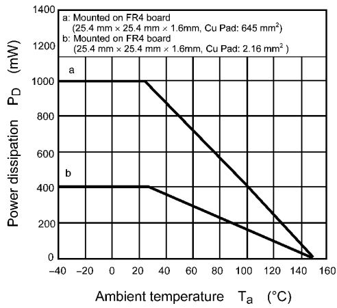
Fig. 7.13 P_D - T_a
